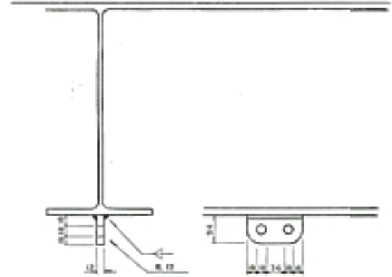
小梁吊り止め用A型A種（又は垂吊用種）
