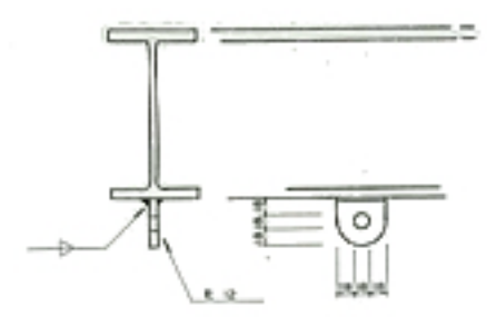
小梁吊り止め用A型A種
