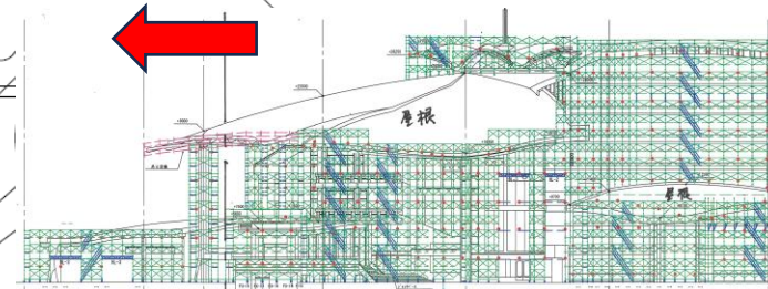
北面立面図
