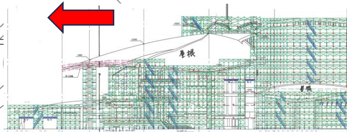
北面立面図
